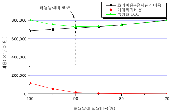
그림 6 허용능력 변화에 따른 주형의 총기대 LCC
