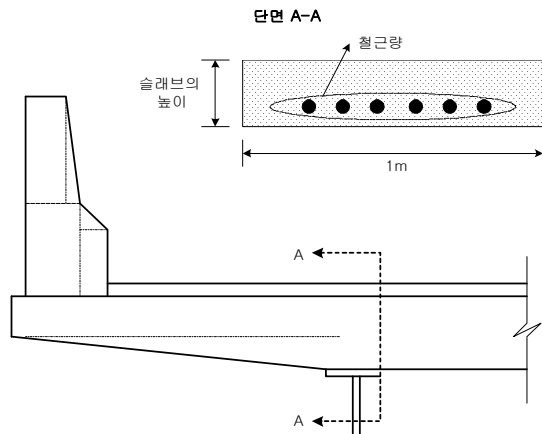
그림 1 바닥판의 설계변수
