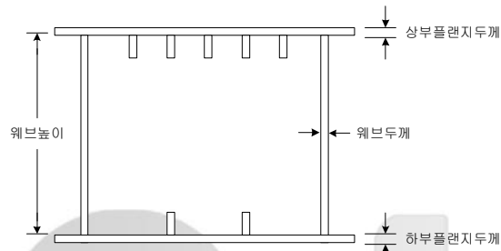
그림 2 주형의 설계변수
