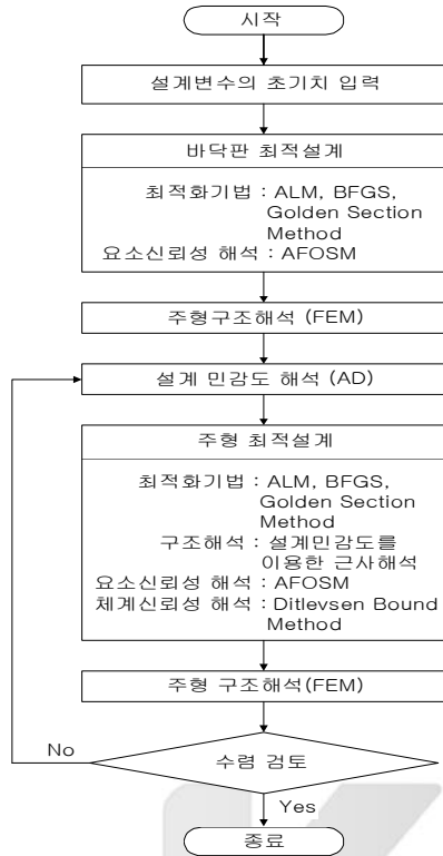
그림 4 강상자형교의 LCC 최적설계 알고리즘
