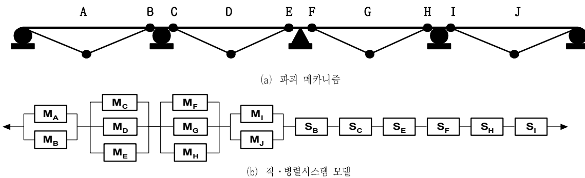
그림 3 체계 신뢰성 해석모델
