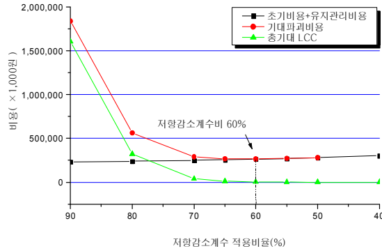
그림 7 저항감소계수 변화에 따른 바닥판의 총기대 LCC
