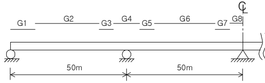
그림 5 종방향 단면그룹
