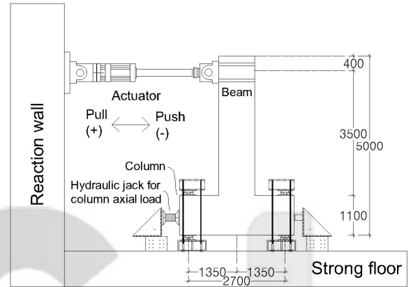
Fig. 2 Test setup
